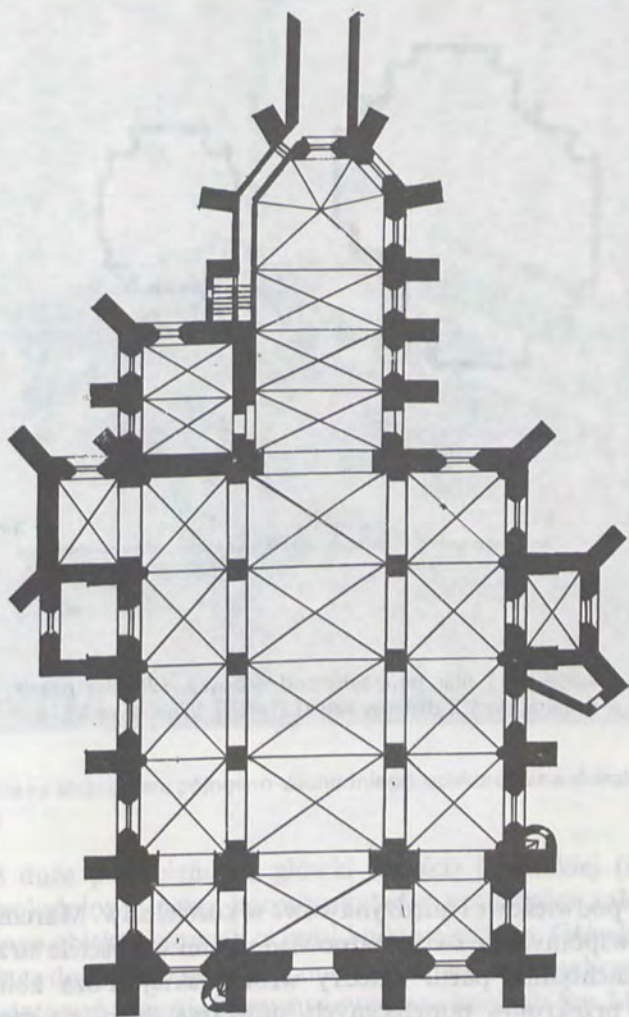
45. Rzut poziomy kościoła Św. Marcina w Jaworze według pomiarów autora i S Kozłowskiego. Skala 1 cm - 5 m
