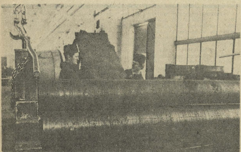
Pracownicy działu montażowego w Przedsiębiorstwie Modernizacji i Remontów wykonują części urządzeń nie tylko dla Celwiskozy, ale dla odbiorców z całej Polski. Na zdjęciu ślusarz-brygadista Adam Romanski i Władysław Moniatowicz przy pracy nad elementami wentylatora dla Zakładu Górniczego Lena w Wilkowie.
