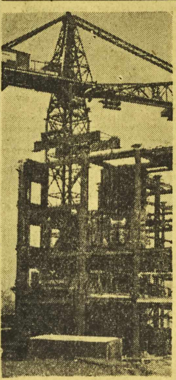
BUDOWE części wysokościowej Pałacu Kultury i Nauki obsługują 4 specjalne dźwigi petające typu UBK-10. Najważniejszą zaletą tych dźwigów jest zdolność samoczynnego podnoszenia się w miarę wzrostu budowy. Na zdjęciu: Fragment dźwigu podniesionego na wysokość pierwszej kondygnacji. CAF — DKN Martynow
