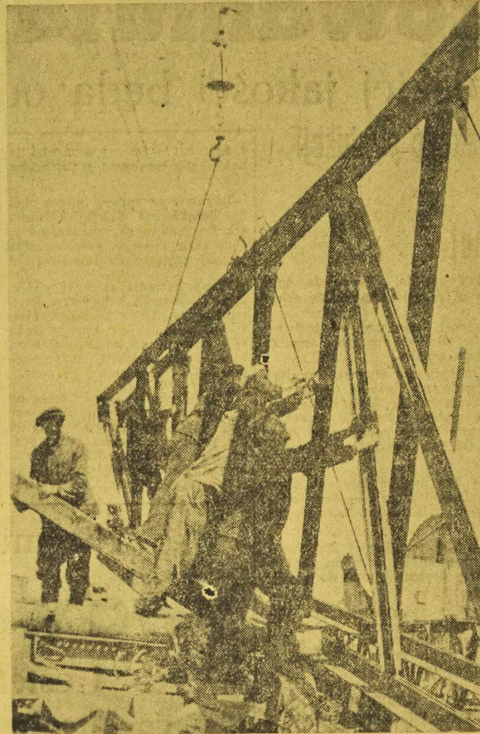
Budowa wielkiej inwestycji Planu 6-letniego, cementowni „Wierzbica“ postępuje szybko naprzód. Na zdjęciu: produkująca brygada montażowa Jana Masteja montuje więzania hali głównej. (CAF — fot. Banduch)
