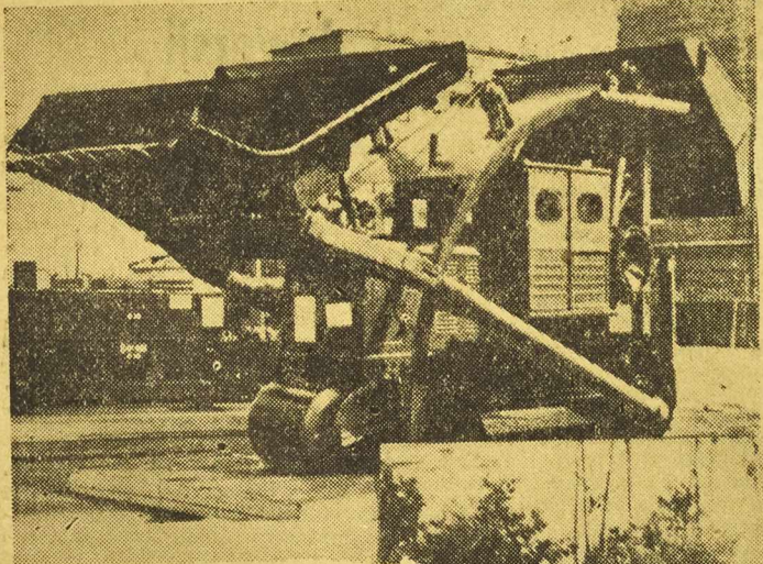
Nasze zdjęcie górne przedstawia ładowarkę traktorową T-107 o pojemności 4,0-6,0 m sześciennych, znajdującą się na wszechwiązkowej stacji wystawie budowlanej w Moskwie.
