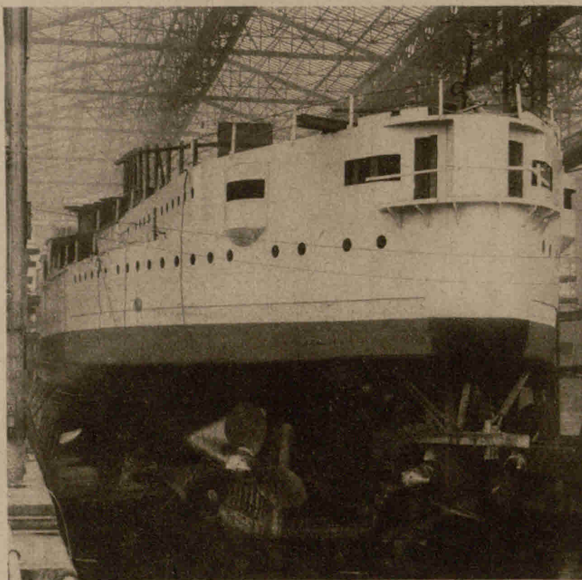
Fertig zum Stapellauf auf der mit Schmierseife eingeschmierten Bahn
