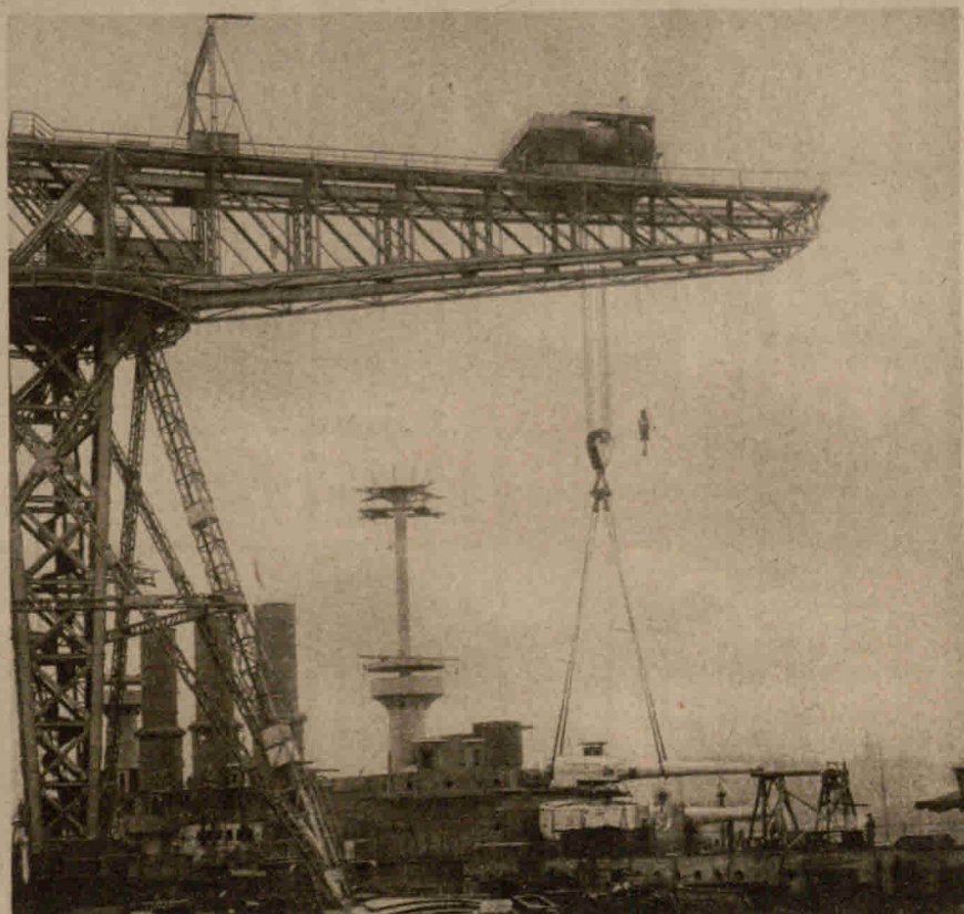
Auf die gleiche Weise wie die Gefechtsmasten werden die Geschütze eingefest
