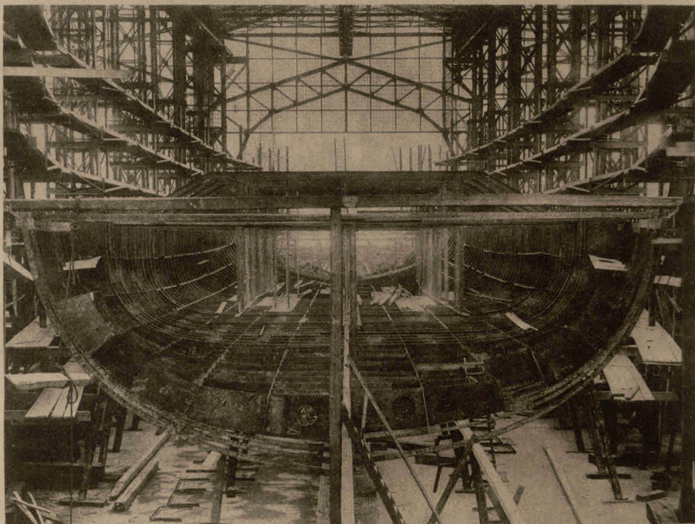
Linien Schiff im Bau, zum Teil in den Spanten stehend
