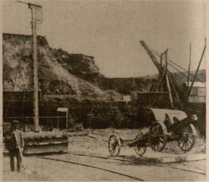
Festigkeitsproben bei der englischen Feldartillerie. Eine schwere Haubise muß mit heftigem Ruck über einen starken Balken hinweg. Als Zugmittel dient ein besonders dafür eingerichtetes Eisenbahnwagen-Gestell
