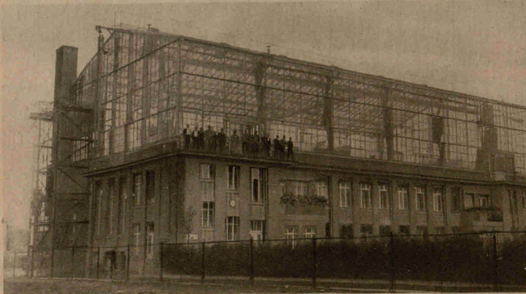
Bild 1. Der Riesenbau einer modernen Filmfabrik, der in der Hauptsache einen gewaltigen Glaskasten in eiserner Umrahmung darstellt
