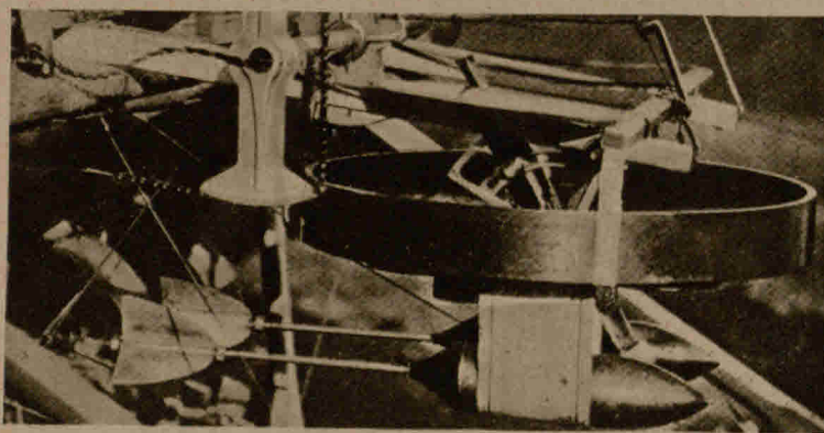
Bombenabwurfvorrichtung an englischem Aeroplan
