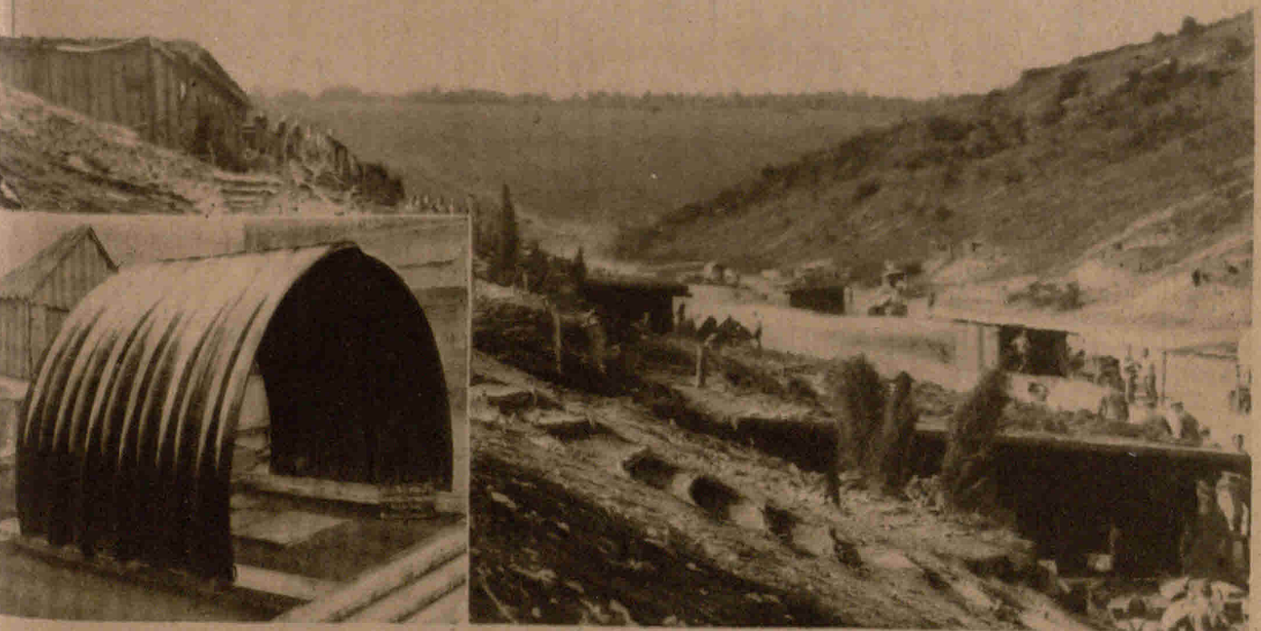
Links: Schutzbücher aus Stahlblech, die in die französischen Schützengräben eingebaut werden. Rechts: In die Felsanhänge der Côte Lorraine eingebaute deutsche Unterstände, bei St. Mihiel *
