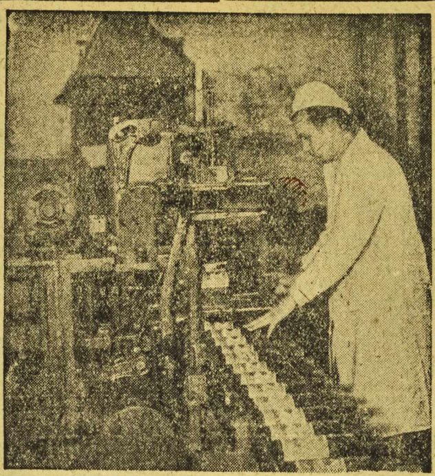
Państwowe Dolnośląskie Zakłady Winiarskie w Legnicy przedterminowo wykonały roczny plan produkcyjny, mimo, że był on o 40 proc. wyższy niż w roku ubiegłym. — Na zdjęciu: Alfred Kocias obsługuje stycykietarkę.
