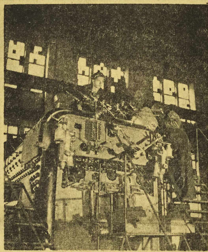
W Zakładach im. Józefa Stalina w Poznaniu produkuje się parowozowy. Na zdjęciu spawacz Andrzej Wiśniewski wyrabiający średnio 150 proc. normy, spawa tablicę amnometrowa. CAF — fot. Baranowski
