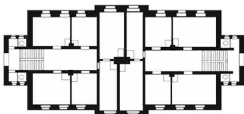
Ryc. 28. Rzut piętra domu czternastorodzinnego. Źródło: opracowanie własne na podstawie materiałów archiwalnych.
