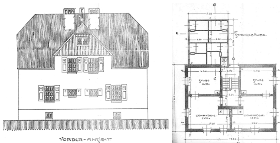
Ryc. 60-61. Projekt domu na osiedlu górniczym przy ul. Piasta. Źródło: WAPK, Akta gm. Biały Kamień, 26, b. s., Zeichnung zum Neubau für Vier-Familien für die Verwaltung der Steinkohlen-Bergwerke Cons. Fuchs. David Grube Hochwaldstr., angrp. Schweidnitz 1914.
