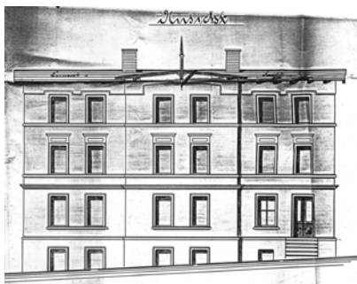
Ryc. 35. Projekt elewacji budynku wielorodzinnego na osiedlu przy ul. Zachodniej w Sobiecinie. Źródło: WAPK, Akta gm. Sobiecin, 544, b. s., Zeichnung zum Neubau eines Wohnhauses für den Berginvaliden Herrn O. Hervig zu N. der Hermsdorf (Feldhammers Grenze) auf seinen Grundstück Hyptk. No 57 Sasselbstr. , W. Köhler, Mauermstr., 1896.
