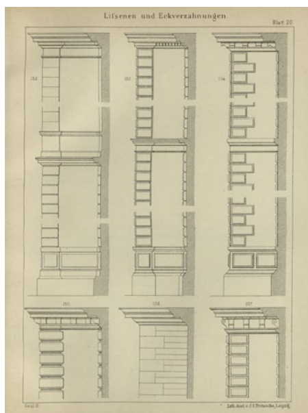
Ryc. 38-39. Boniowania narożne z wzornika, A. Geul, Das Äußere... , Bl. 20, Auf.3, BPK. Przykłady rozwiązań w rejonie wałbrzyskim przy ul. Daszyńskiego nr 29 i narożnik przy ul. Kolejowej nr 16 w Boguszowie. Fot. Bogna Ludwig. Źródło: archiwum Autorki.
