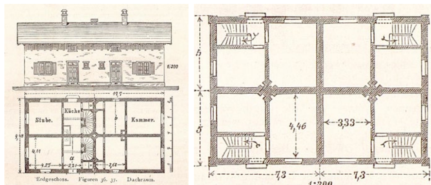
Ryc. 31-32. Domy poczwórne osiedla kolejarskiego w Marburgu, rzut poddasza i elewacja frontowa oraz domu osiedla spółdzielni w Liège (Lüttich), rzut parteru. Źródło: L. Klasen, Die Arbeiter... , s. 40, 43. Köln, ZB MED.-Informationszentrum Lebenswissenschaften 2017, urn:nbn:de:hbz:38m:1-32923.
