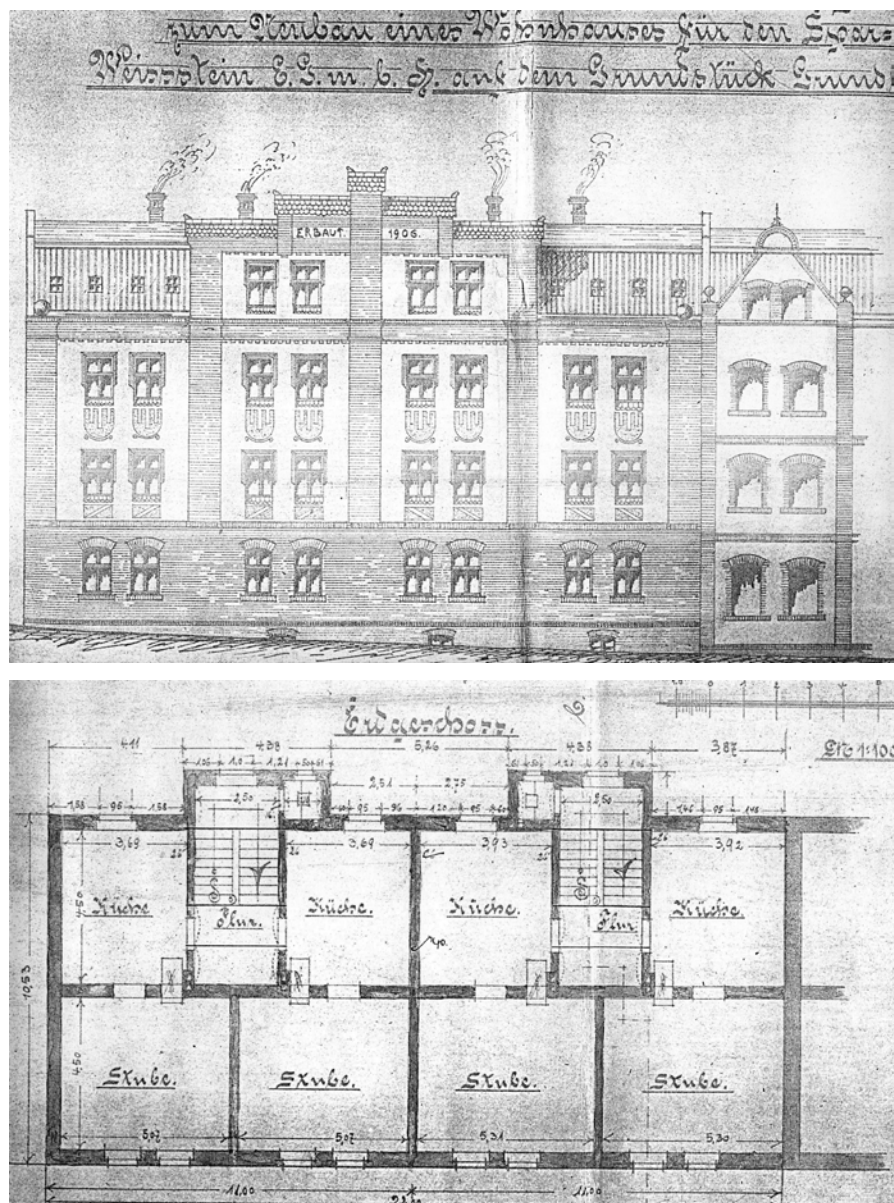
Ryc. 44-45. Projekt elewacji i rzut parteru kamienicy przy ul. Reja 24. Źródło: WAPK, Akta gm. Biały Kamień, nr 24, s. 95, Zeichnung zum Neubau eines Wohnhauses für den Spar- und Bauverein GmbH auf dem Grundstück Grundbuch Blatt 325/326 in Weissstein, M 1:100, Mauermeister J. Schiedock, Bauer. H. Hoffmann i G. Hoffmeister, zatw. 4 Feb. 1906.
