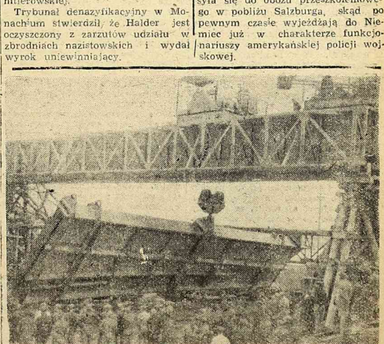
PIERWSZE PRZEŚŁO MOSTU ŚLASKO-DĄBRÓWSKIEGO DZWIGA ONZ W GOŃE
