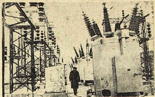
Nad rzeką Syr Daria w Farkhad w Uzbekistanie trwają obecnie prace końcowe przy budowie wielkich zakładów elektrycznych. Na zdjęciu: zespół transformatorów
