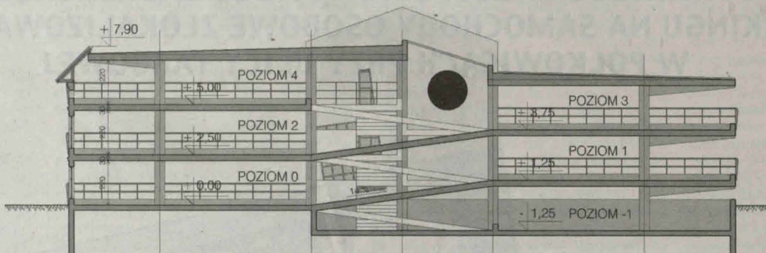
PRZEKRÓJ A - A SKALA 1 : 100
