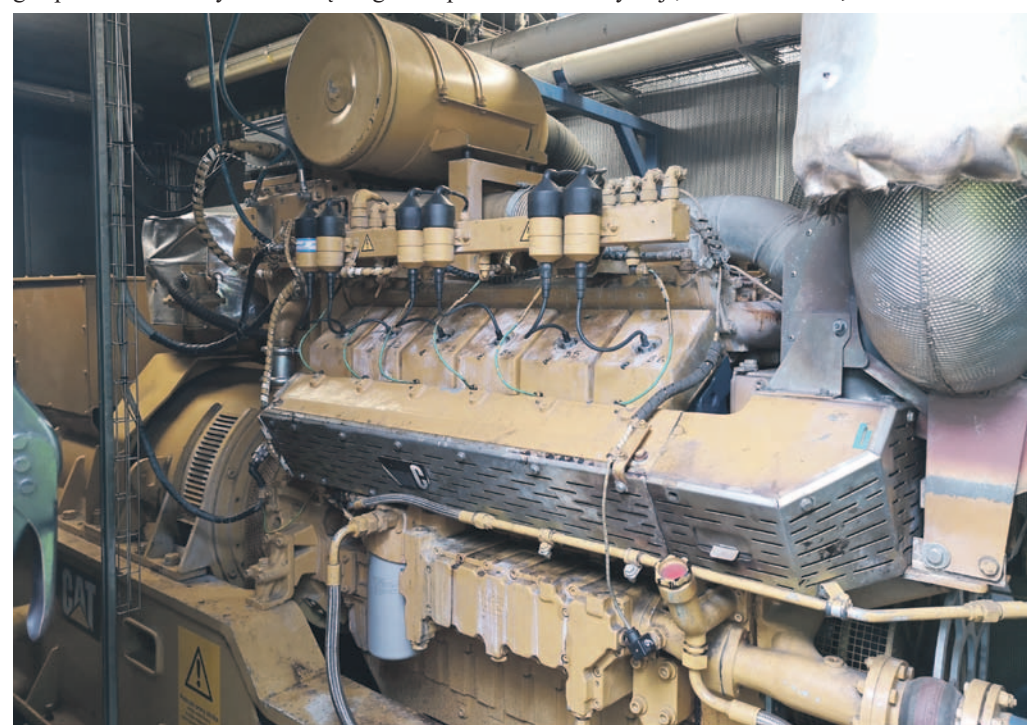
Tu są dwie jednostki kogeneracyjne, czyli silniki gazowe, sprzężone z turbiną elektryczną, produkującą prąd
