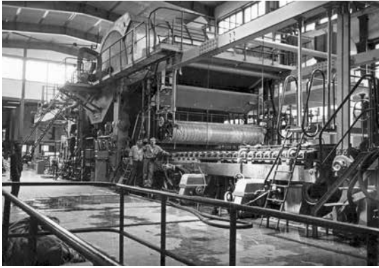
Ryc. 32. Ta maszyna postawiona w Izmir w Turcji, mogła już na klientach robić wrażenie...
