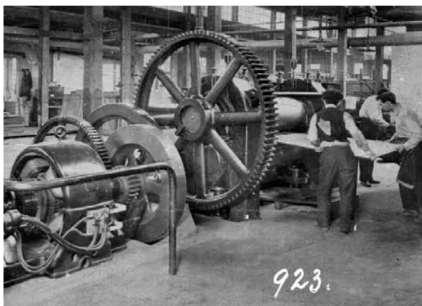
Ryc. 12. Na początku XX wieku maszyny miały już napęd elektryczny
