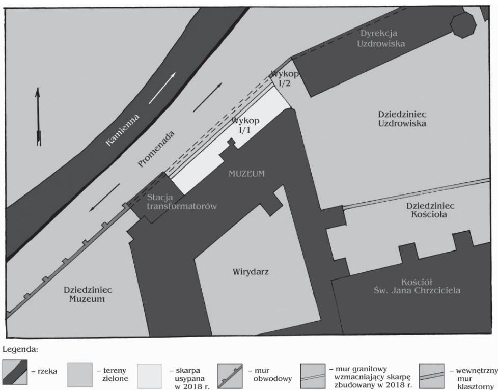
Jelenia Góra - Cieplice dz. 59/11, 59/12. Lokalizacja wykopów badawczych I/1 i I/2. Skala 1:500.
