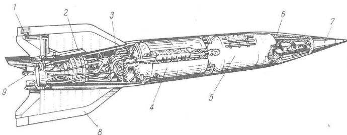
Rakietka V-2: 1 - ster aerodynamiczny, 2 - komora spalania silnika rakietowego, 3 - pompy, 4 - zbiornik ciekłego tlenu, 5 - zbiornik alkoholu, 6 - pilot automatyczny, 7 - głowica z materiałem wybuchowym, 8 - stabilizatory, 9 - grafitowe ster gazodynamiczne
