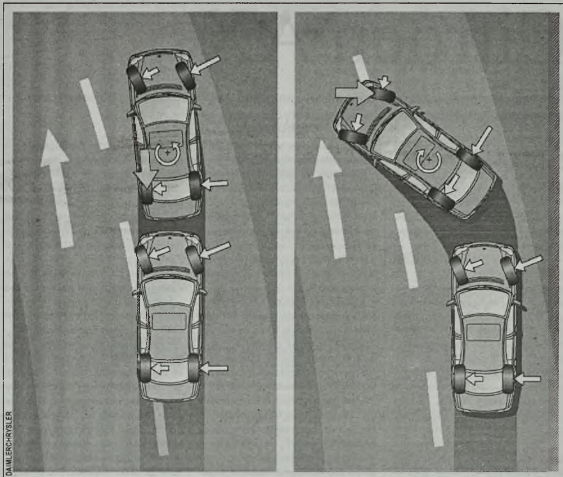
System ESP sprawia, że samochód utrzymuje swój tor jazdy. Podczas podsterowności (grafika po lewej) przednie koła skręcają na zewnątrz – wtedy ESP automatycznie wyhamowuje lewe tylne koło. Podczas nadsterowności (grafika prawa) ESP hamuje prawym przednim kołem
