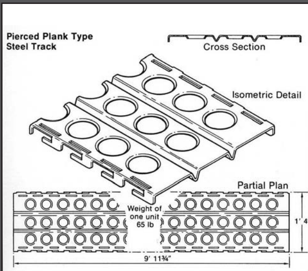
Panel PSP (Pierced Steel Plank „Marston” oznaczenie wojskowe M 8), miał następujące rozmiary: długość 3 metry (10 stóp dokładnie 9, 11 cali 3/4) szerokość 38 cm (1 stopa 4, 15 cali) w jednym panelu - 29 otworów (odwadniających) w trzech rzędach a więc całość miała 87 otworów.
