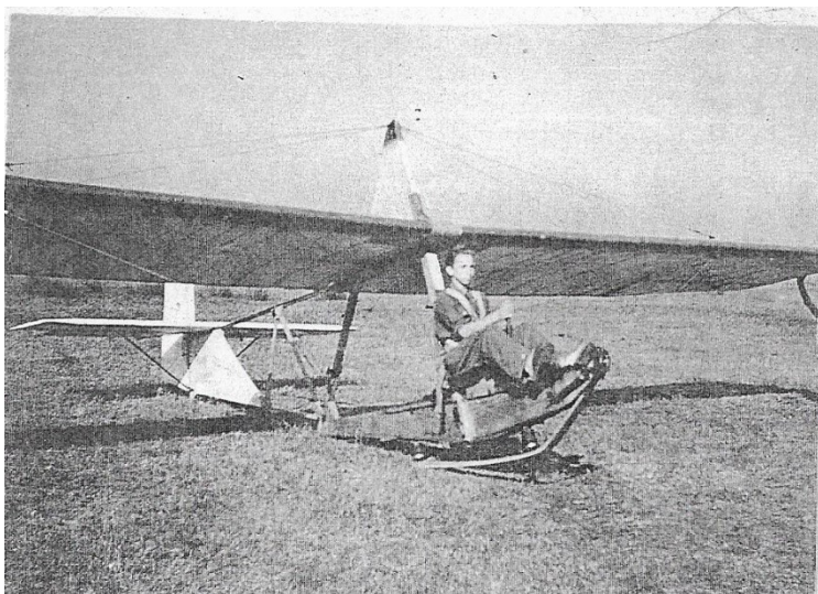
Szybowiec SG-38
