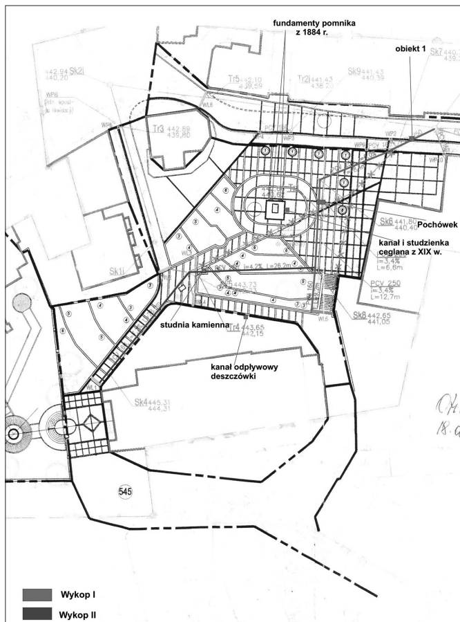
Ryc. 5. Projekt rewitalizacji przestrzeni publicznej placu Kościelnego w Wałbrzychu z zaznaczonym przebiegiem wykopów i odsonionymi obiektami, skala 1:500
