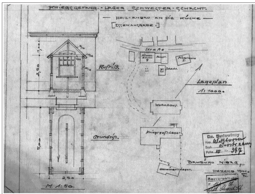
Ryc. 5. Plan obozu dla jeńców wojennych na terenie szybów siostrzanych – lager Schwesternschacht Źródło: AMGR, sygn. 16 K
