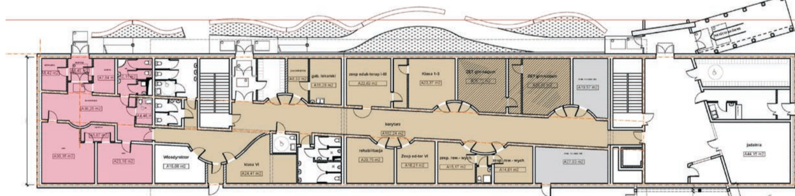
Rzut parteru nowej placówki oświatowo-opiekuńczej
