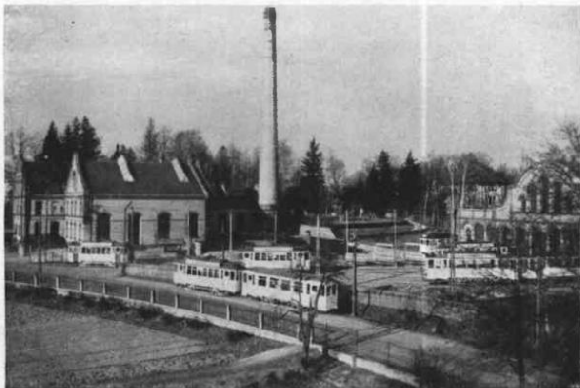
Kraftwerk Hirschdorf der Hirschberger Thalbahn A.-G.
